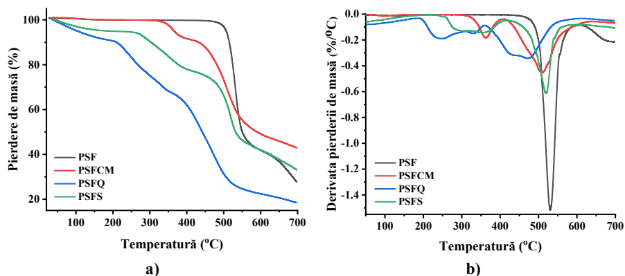
Figura 2.14. Curbele a) TG și b) DTG înregistrate pentru polisulfona nemodificată și polisulfonele funcționalizate cu grupările: clorometil ( PSFCM ), clorură de dimetilbutilamoniu ( PSFQ ) și \text{SO}_3\text{H} ( PSFS )
